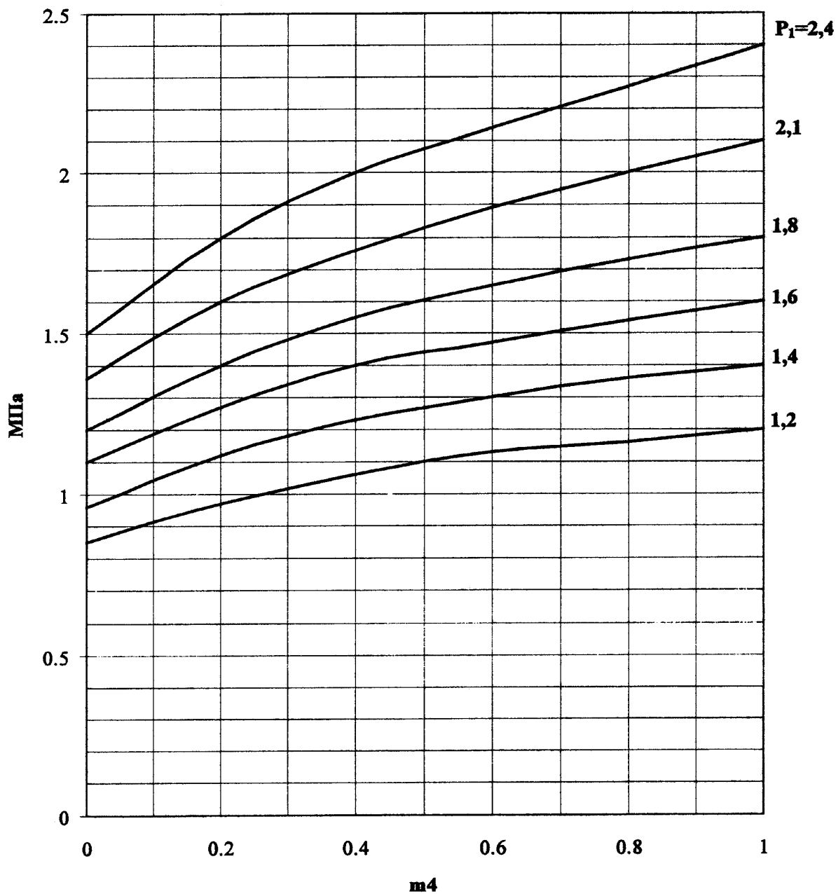
График для определения давления в изотермическом резервуаре в конце выпуска расчетного количества двуокиси углерода
